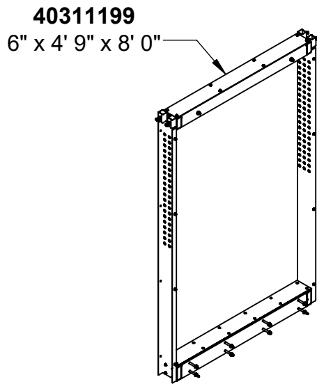
Cage extension 6" (Extension de cabine 6")
