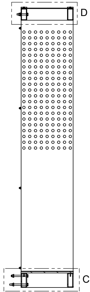
SECTION A-A
