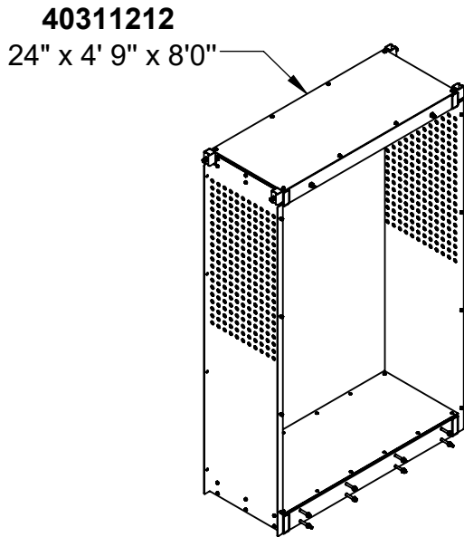
Cage extension 24" (Extension de cabine 24")
